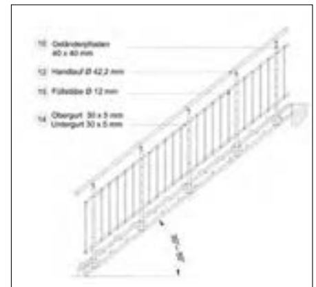
Geländervariante Typ S
