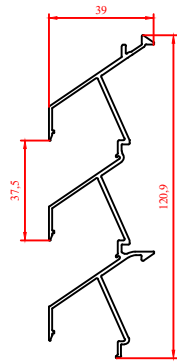
DWS Dreifachlamelle 30Z NP P1177110
