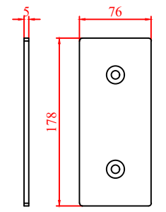
Abdeckplatte der Klaue G0105201
