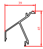
DWS Lamelle 30Z NP P1184210
