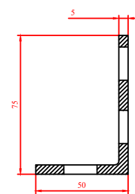
L - profil 75/50/5 T1121510
