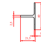
DWS Halteprofil 40/21 T1195010
