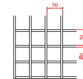
Galva Netze 1350x2750, Gewinde Ø 6mm, Maschenweite 50x50 G0105200
