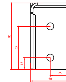
Verstärktes Edelstahl L-Profil 85/85/3 G0105408
