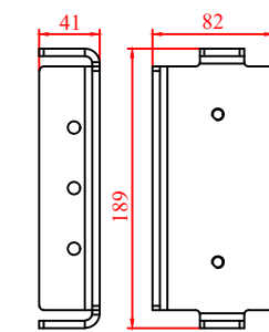
Einbruchhemmende Klaue G0105202
