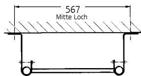
Wandbefestigungen nach außen montiert
