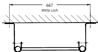
Wandbefestigungen nach außen montiert
