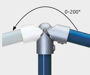
Best.-Nr. 0520 1500 00 Winkelgelenkstück Verstellbereich 0° – 200°. Einsetzbar anstelle von Rohrbiegungen.
