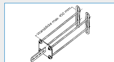
Für 1 Wandanschluss teil mit 4 Bohrungen (2 Sätze notwendig)
