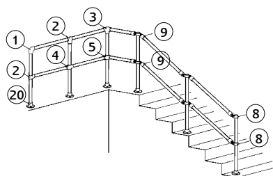
Treppen- und Podestgeländer
