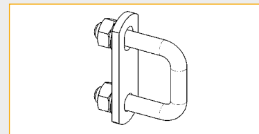
Bügelschrauben – eckig, Typ 0529.85.40
