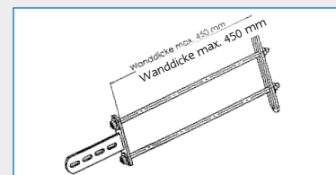
Für 1 Wandanschluss teil mit 2 Bohrungen (1 Satz notwendig)
