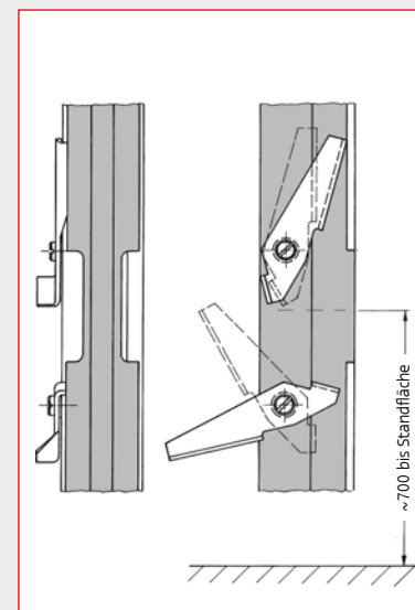
Ausklinkung mit Endanschlüssen
