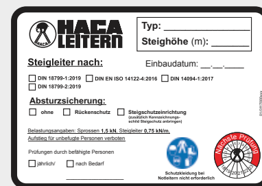
Typ 0173.10 / Typ 0174.10 Kennzeichnung der Klasse des Anwenders nach DIN 18799:2019
