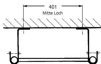
Wandbefestigungen nach innen montiert
