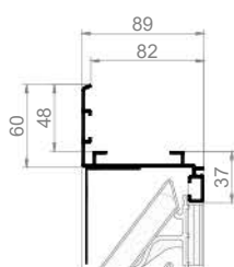
G 75Z Einbauwandgitter mit Flansch
