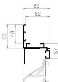
G 50HP Einbauwandgitter mit Flansch
