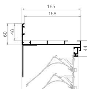
G 130HP Basic Einbauwandgitter mit Flansch
