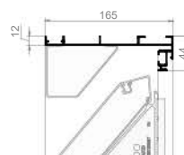
N 150 Einbauwandgitter ohne Flansch
