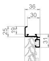
G 20V Einbauwandgitter mit Flansch
