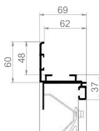
G 50Z Einbauwandgitter mit Flansch
