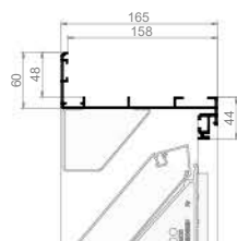
G 150 Einbauwandgitter mit Flansch
