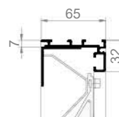
N 50/75Z Einbauwandgitter ohne Flansch
