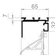
N 50HP Einbauwandgitter ohne Flansch
