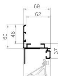
G 45HP Einbauwandgitter mit Flansch
