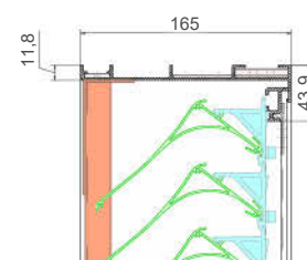
N 130HP Einbauwandgitter ohne Flansch
