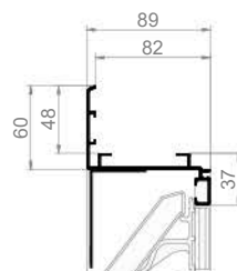
G 75L Einbauwandgitter mit Flansch
