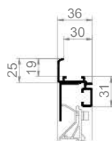
G 20Z Einbauwandgitter mit Flansch
