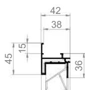
++ G 30Z Einbauwandgitter mit Flansch
