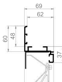
G 50/75Z Einbauwandgitter mit Flansch
