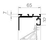
N 45HP Einbauwandgitter ohne Flansch
