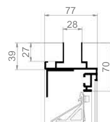
F 45HP Lüftungsgitter für Fenster
