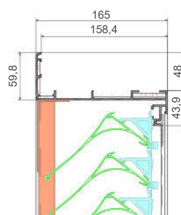
G 130HP Einbauwandgitter mit Flansch
