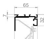
N 50Z Einbauwandgitter ohne Flansch
