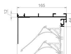
N 130HP Basic Einbauwandgitter ohne Flansch
